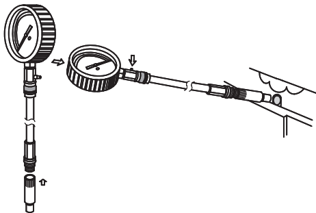
Рисунок 6. Присоединение через резьбовой адаптер.
